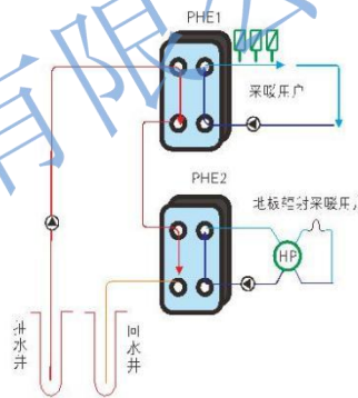
板式换热器在地热系统中的应用
