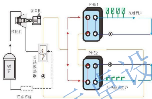
板式换热器在集中供热系统中的应用
