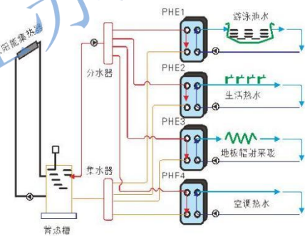
板式换热器在太阳能集热系统中的应用
